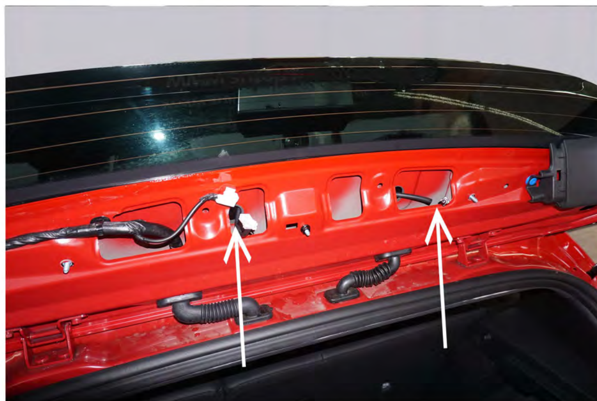
Kabelstecker und Schlauch lösen.
